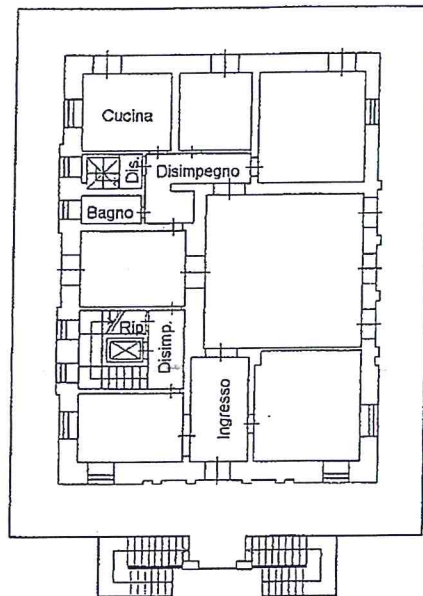
Pianta Piano Terra H= mt. 4.70
